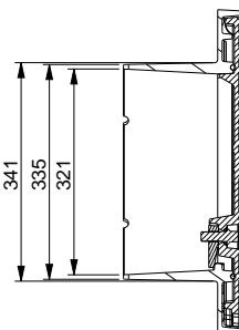
COUPE A-A
