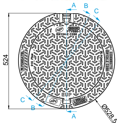
Position basse A-A
