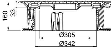
Encoche 1 B-B
