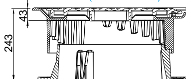
Encoche 8 (Position haute) A-A
