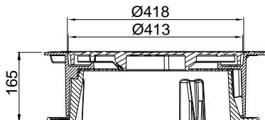
Encoche 1 B-B
