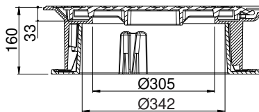
Inkeping 1 B-B
